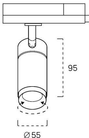
Рис.4-5. Габаритные размеры светильников
