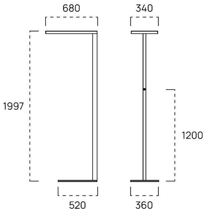
Рис.2. Габаритные размеры светильников
