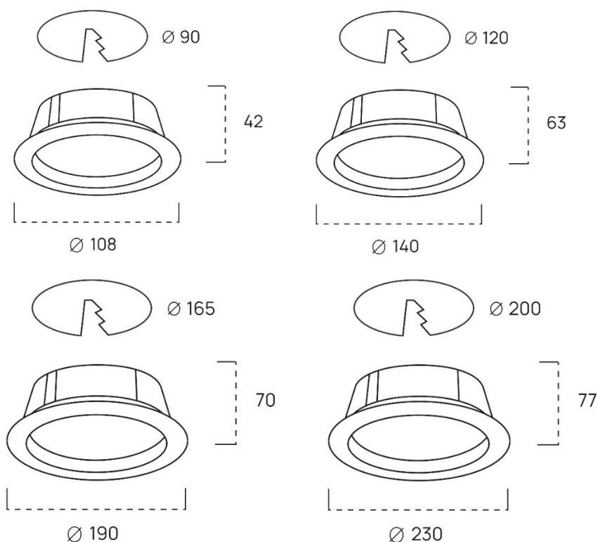
Рис.2-5. Габаритные размеры светильников
