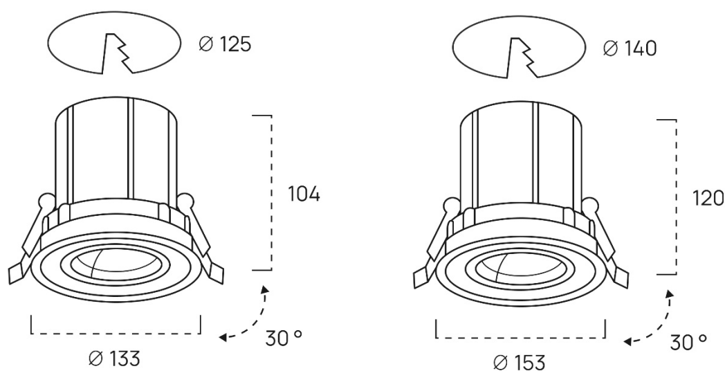
Рис.2-3. Габаритные размеры светильников
