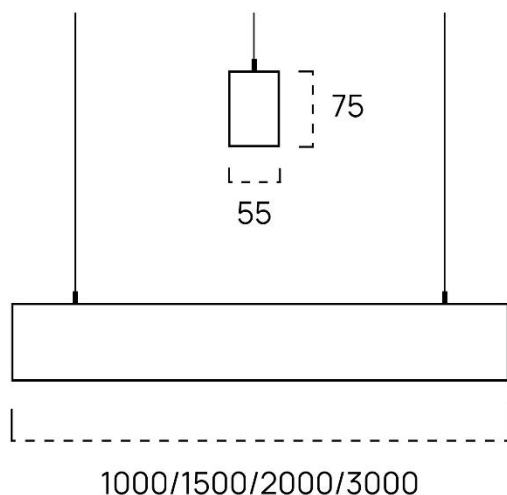
Рис.2. Габаритные размеры светильников
