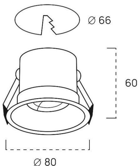
Рис.3. Габаритные размеры светильников
