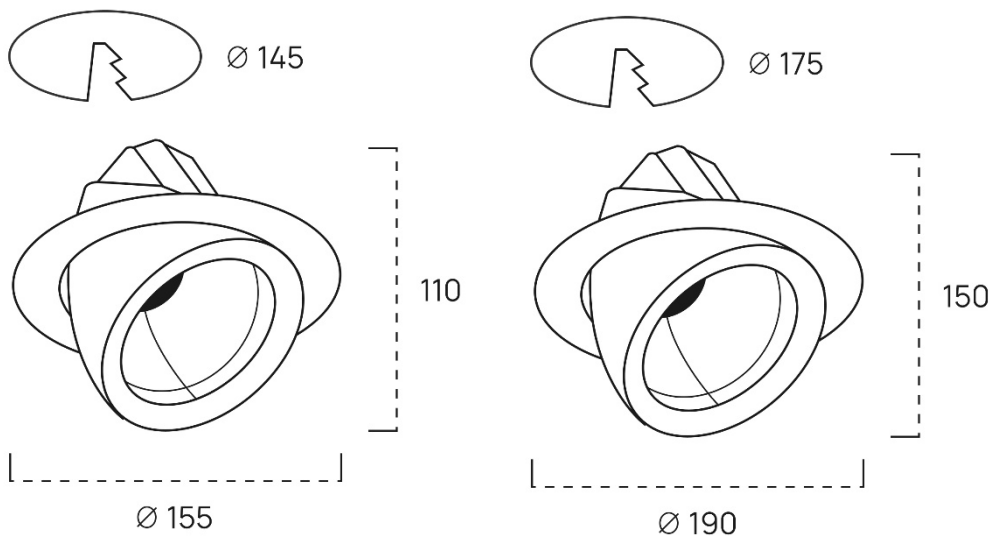
Рис.2. Габаритные размеры светильников
